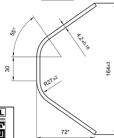
Schnitt A-A
