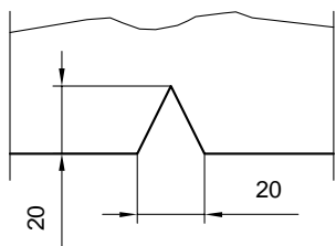
Einzelheit W
