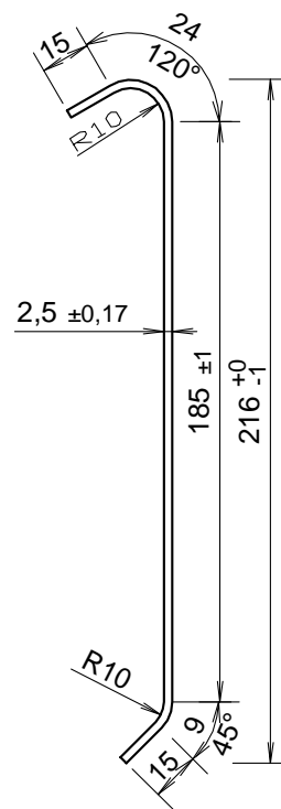
Schnitt B-B
