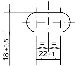
Einzelheit Y
