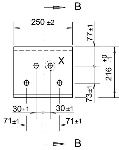
Teil Nr. 23.10
