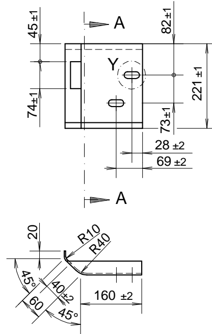
Teil Nr. 23.20
