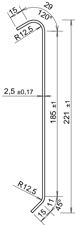
Schnitt A-A
