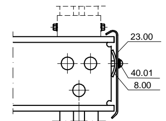
Einzelheit X
